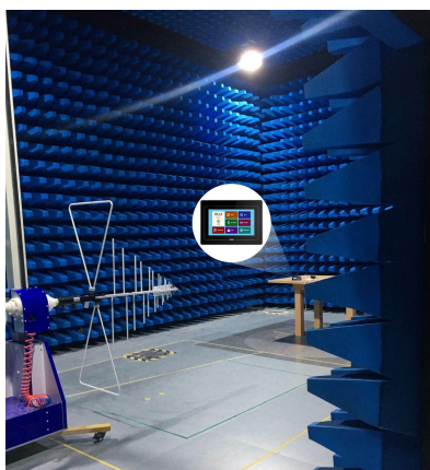
图 5-4 RE 测试图
