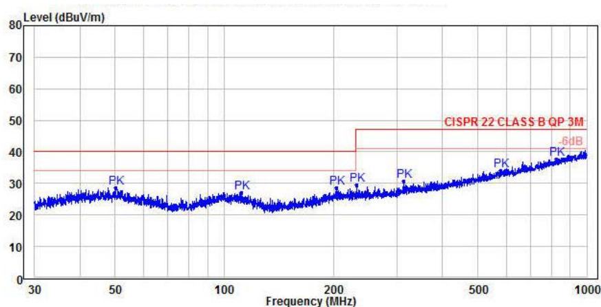
图 5-5 RE 测试水平方向
