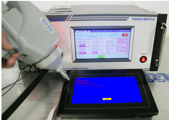
图 5-2 ESD 测试图
