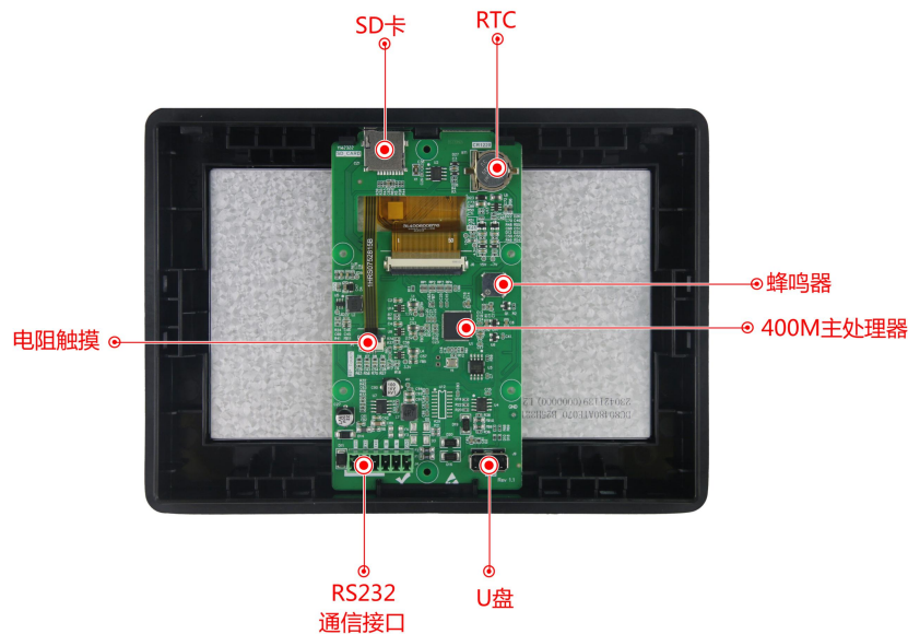
图 1-2 硬件配置图
