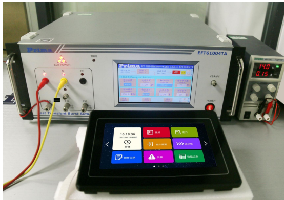
图 5-3 EFT 测试图
