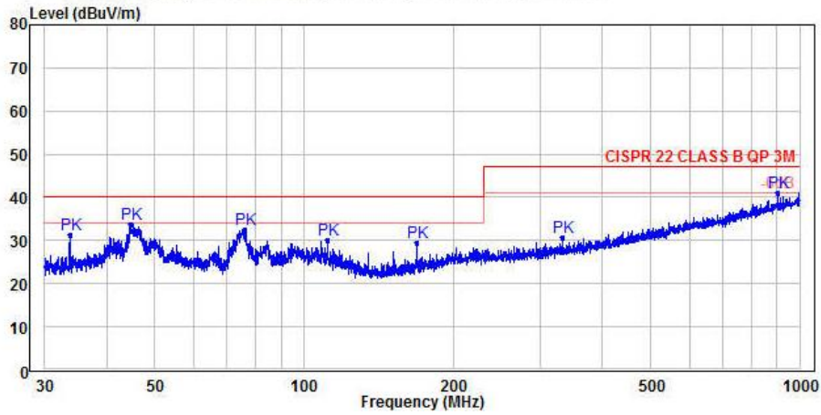
图 5-6 RE 测试垂直方向
